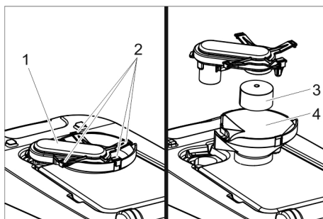
1 Корпус поплавка 2 Фиксирующие крюки
